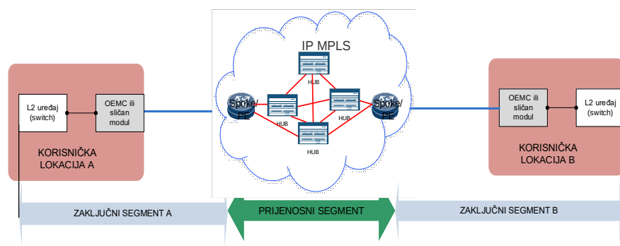
Slika 1. Načelan prikaz E2E realizacije Ethernet voda
