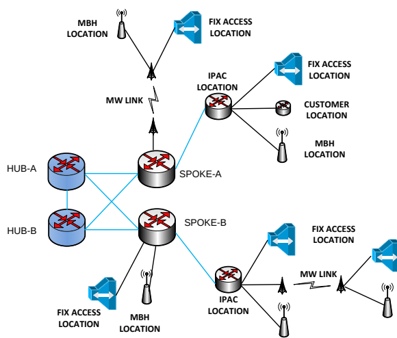
Slika 1.1 Logički prikaz povezivanja elemenata IP MPLS mreže
